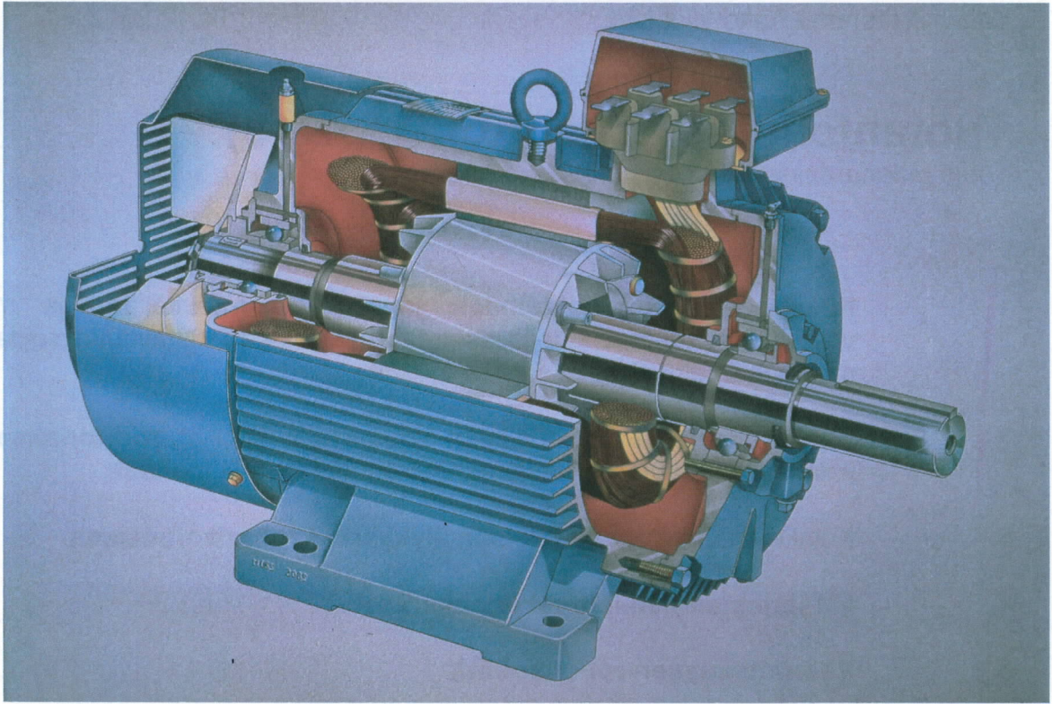
Kuva 1. Sähkömoottori
